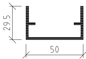
Profil Nr.16250
