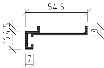
Profil Nr.16248
