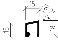
Profil Nr.16249
