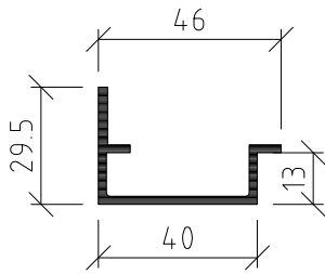
Profil Nr.16247
