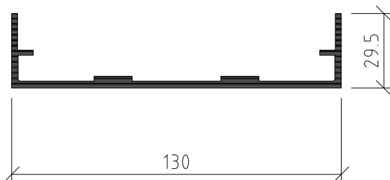
Profil Nr.16251
