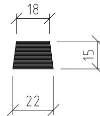
Profil Nr.16246
