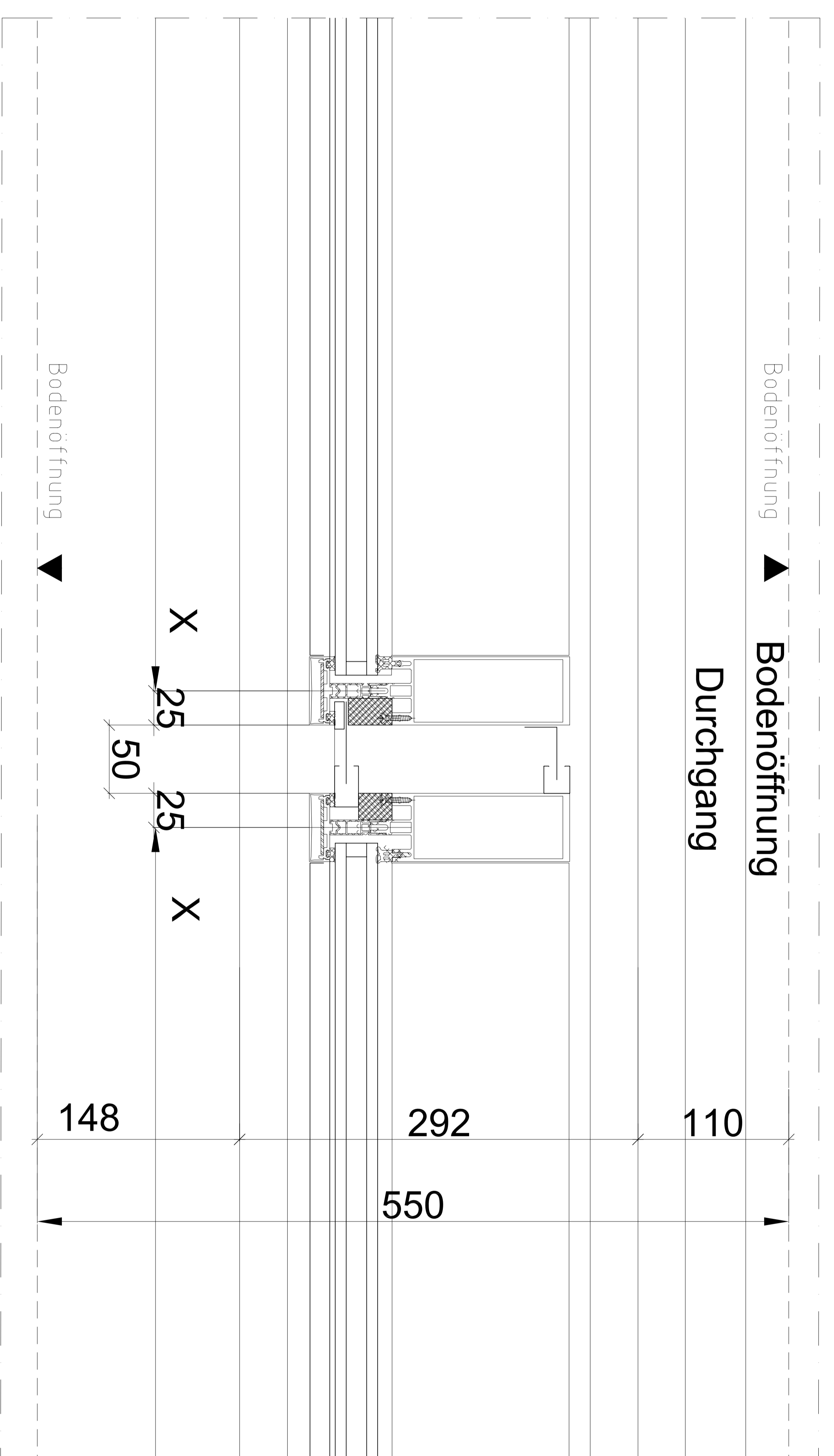
Horizontalschnitt 101-101
