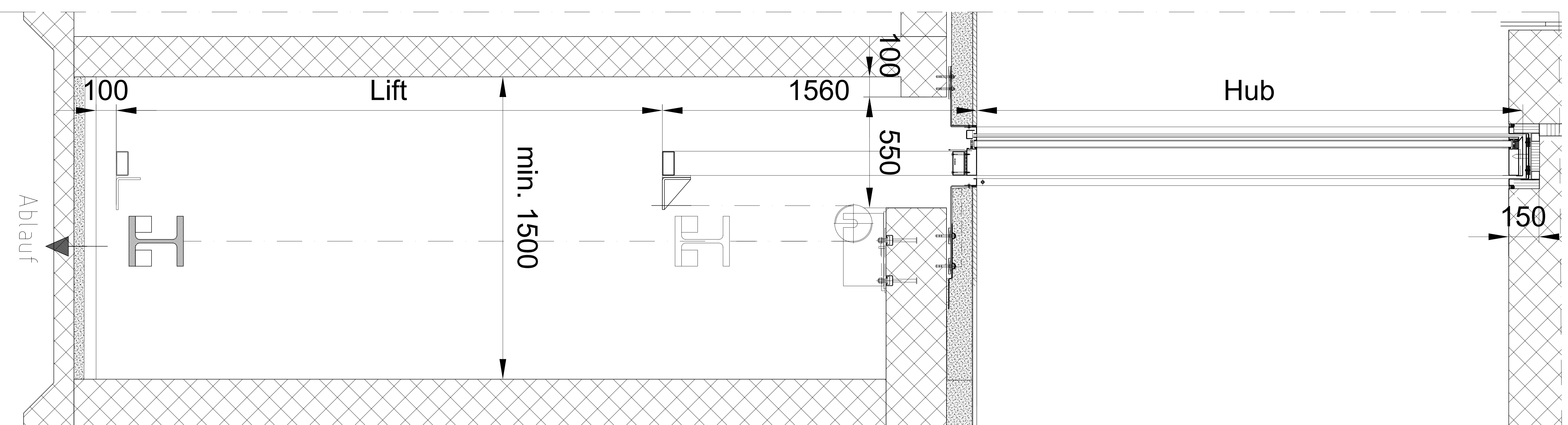
Vertikalschnitt 201-201
